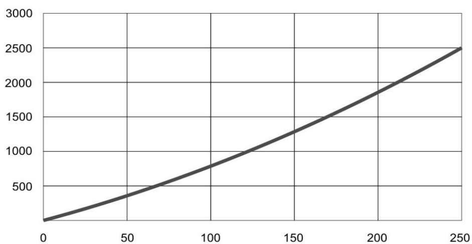
Tabulka tlakové ztráty kolektoru SK12-CPC
