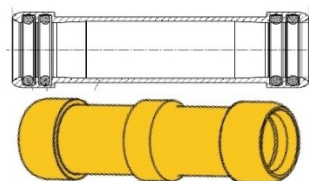
Hydraulická spojka SKR-HV 110050
